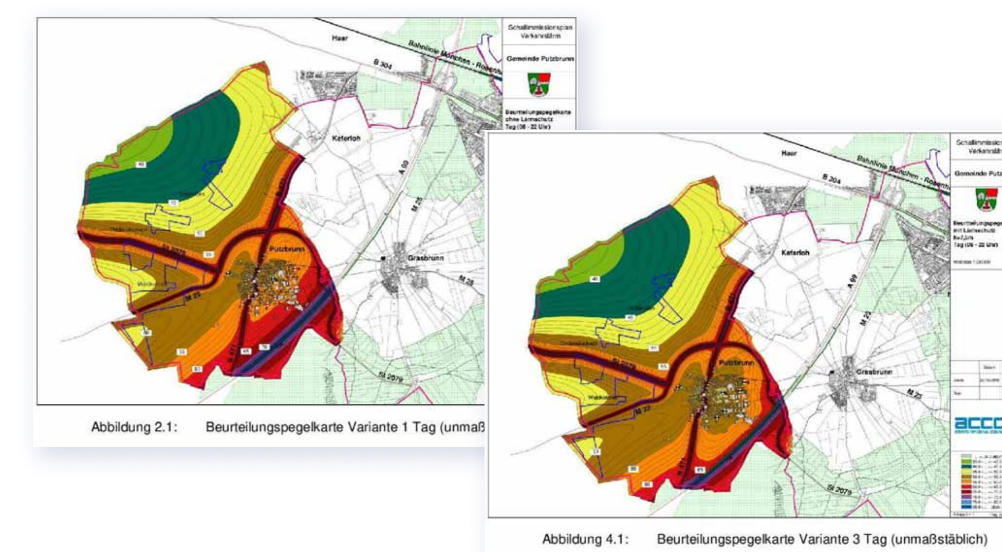
Schallimmissionsplan von Putzbrunn am Tag (links) und mit einer 7,5m hohen Schallschutzwand an der Autobahn (rechts) erstellt durch die Firma ACCON GmbH Okt. 2018.
