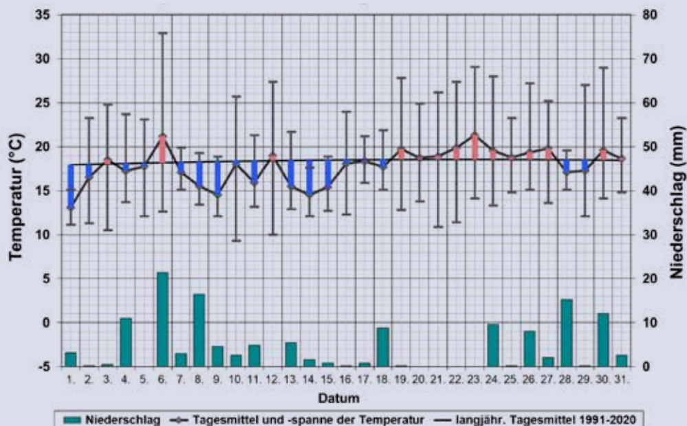
Temperatur und Niederschlag in Putzbrunn im Juli 2021
